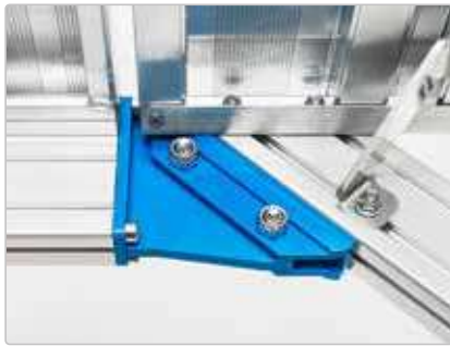
Verbindung Treppe/Plattform
